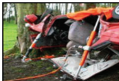
Figura 48: Macacos (permite afastar estruturas que se encontrem mais distantes como, por exemplo, afastar o tablier ou elevar o tejadilho).
